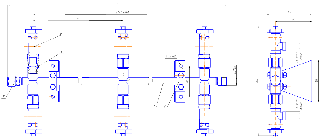
Рис.1 Коллектор рамповый КР-03 ДЖЕТ 304 24 00 00, ДЖЕТ 304 40 00 00 1- коллектор; 2 - кронштейн; 3 - клапан запорный, 4 - переходник; 5 - заглушка.
